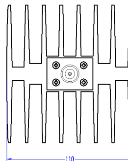
左视图
