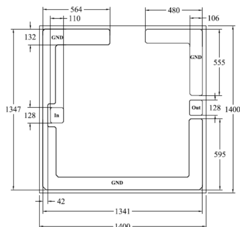
外形结构图 (um)
